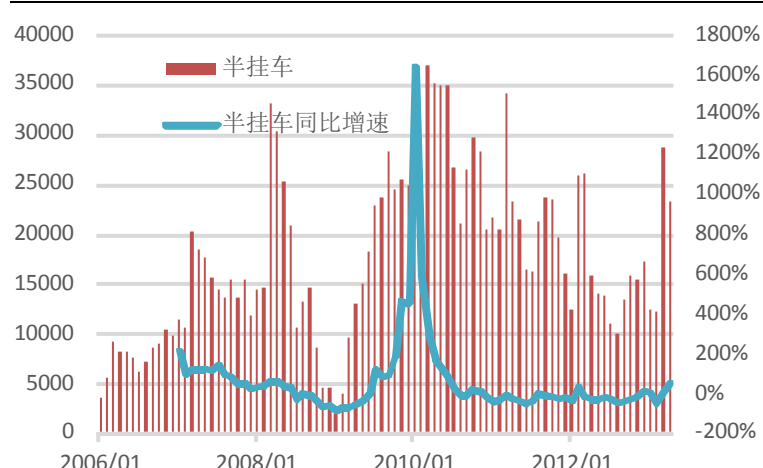
图 32: 半挂车销量
