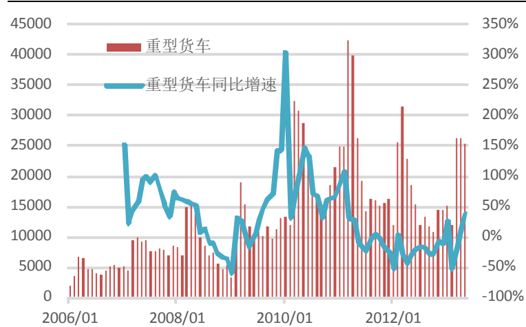
图 28：重货销量
