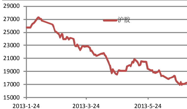
图 1：沪胶走势图
